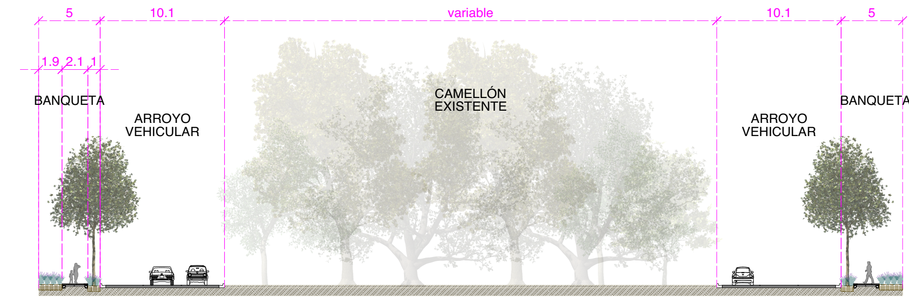
SECCIÓN VIAL TIPO 1:300
